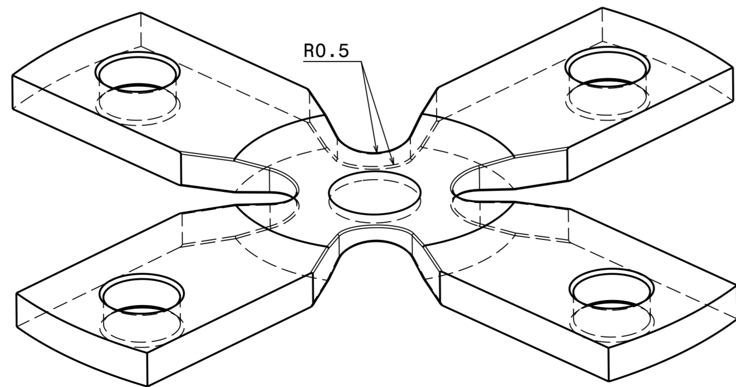
Isometrische Ansicht M 1:1
