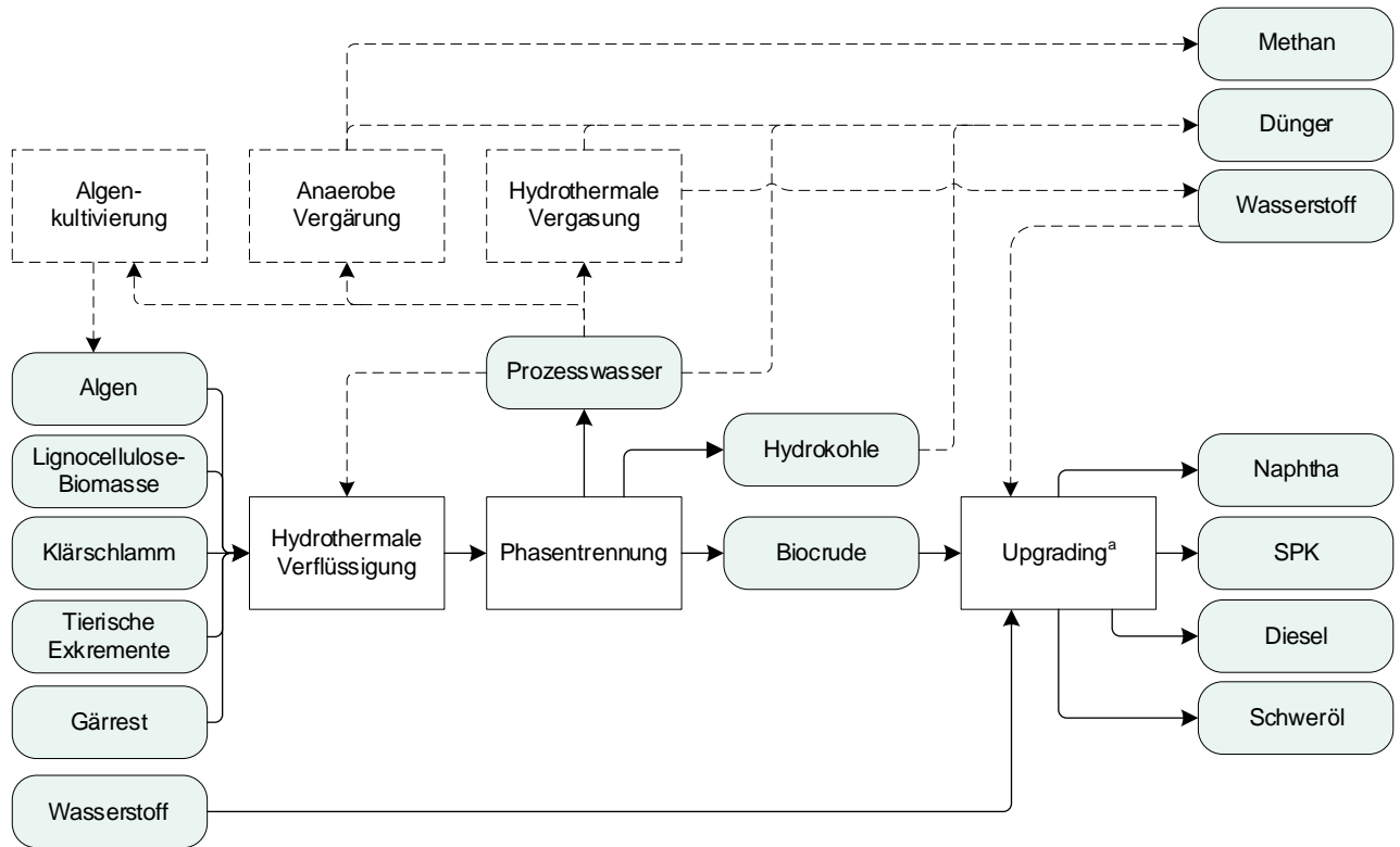
Abbildung 3-8 Schematische Darstellung der Produktion von HTL-Kraftstoffen
