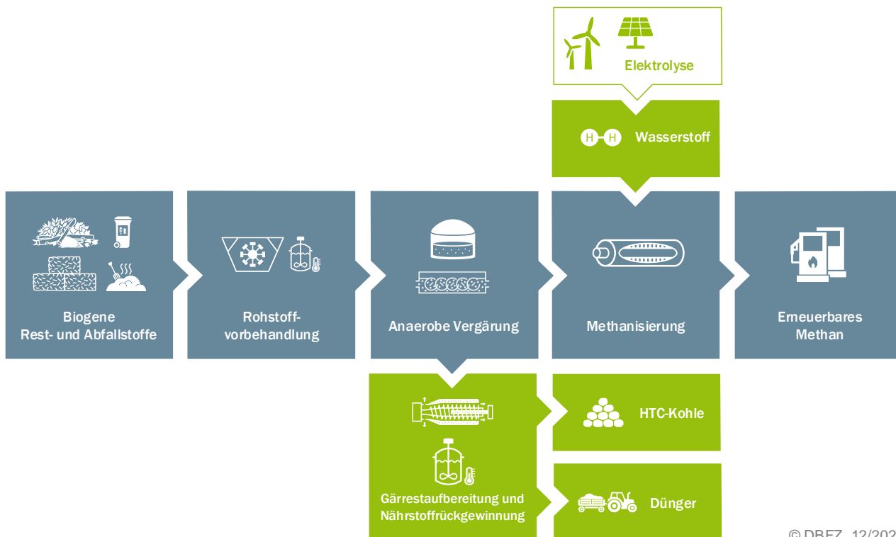
Abbildung 3-16 Prozesslayout für die Pilotanlage des Projekts „Pilot SBG“ Hinweis: keine praktische Umsetzung der Elektrolyse, [DBFZ (2021a)]
