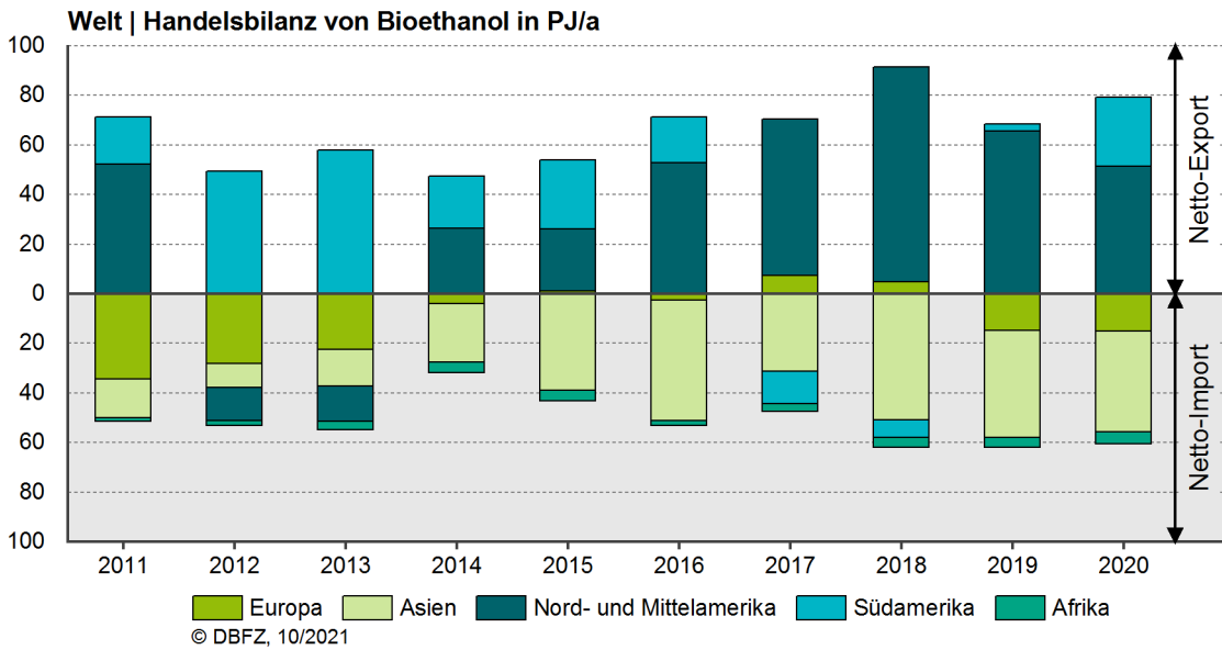
Abbildung 5-15 Bioethanol – weltweite Netto-Handelsbilanzen , Darstellung enthält auch stofflich genutztes Bioethanol, eigene Berechnung auf Datenbasis: [F.O. Licht (2012b), (2015c), (2016c); IHS Markit (2020b)]
